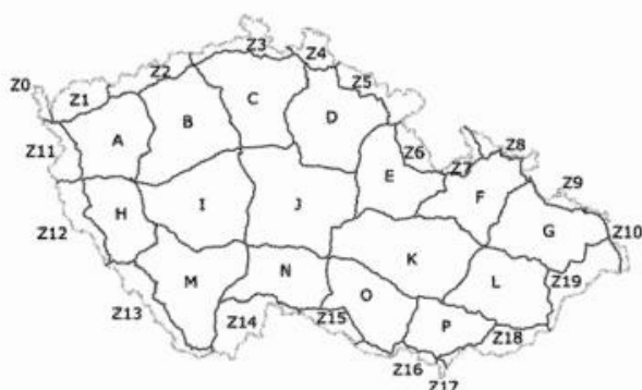
Označení nivelačních oblastí I. řádu
